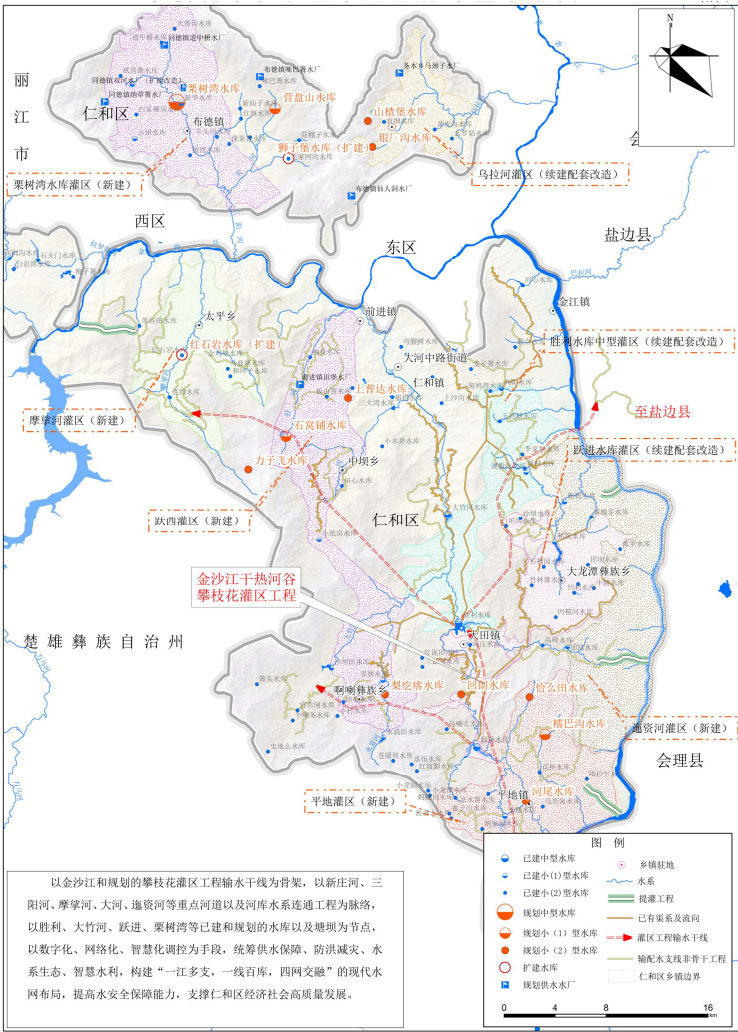
图 2.6- 1 仁和区水网总体布置示意图
